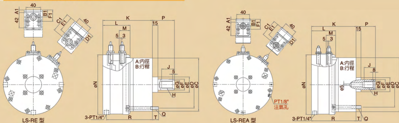
尺寸圖 > Dimensions
