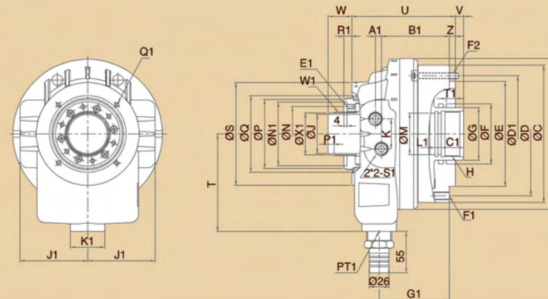
尺寸圖 » Dimensions
