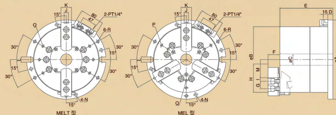
尺寸圖 » Dimensions
