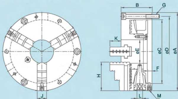
尺寸圖 » Dimensions
