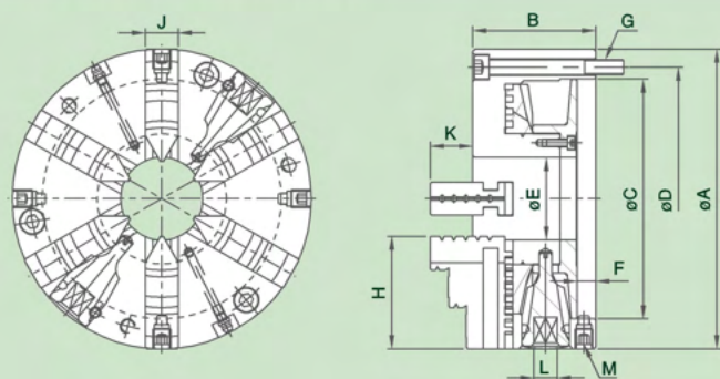
尺寸圖 » Dimensions
