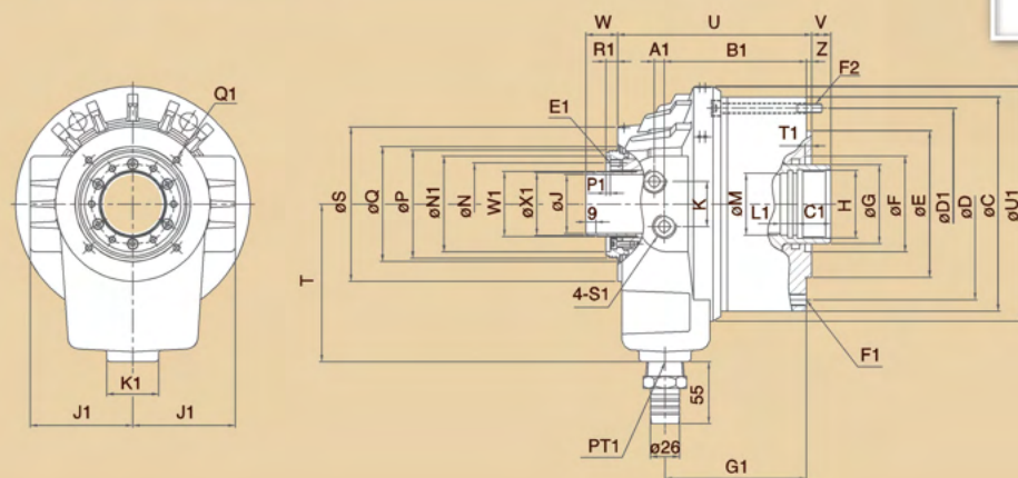
尺寸圖 » Dimensions
