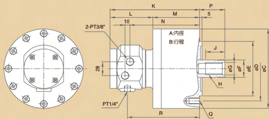
尺寸圖 » Dimensions
