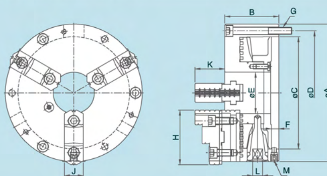
尺寸圖 » Dimensions
