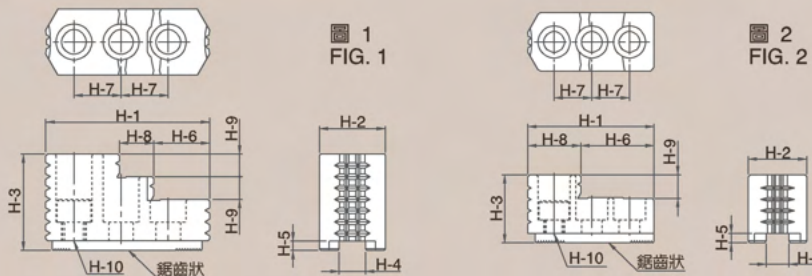
規格表 » Specifications
