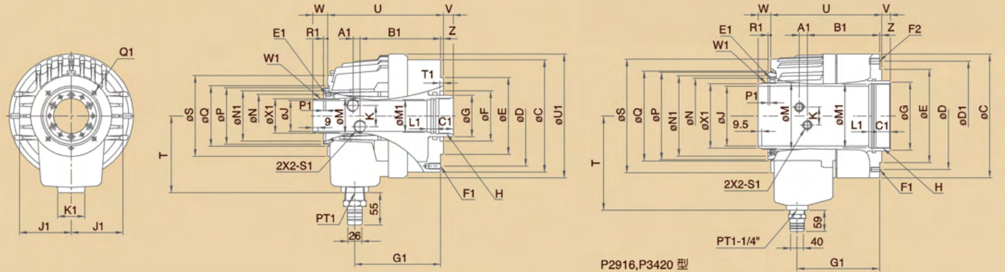
尺寸圖 » Dimensions
