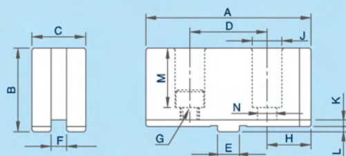
尺寸圖 » Dimensions
