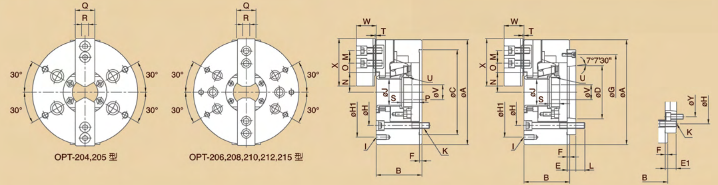
尺寸圖 > Dimensions
