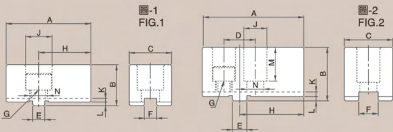
規格表 » Specifications
