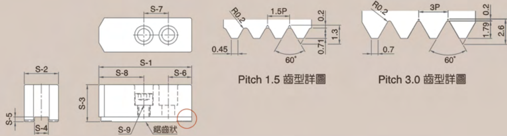
規格表 » Specifications
