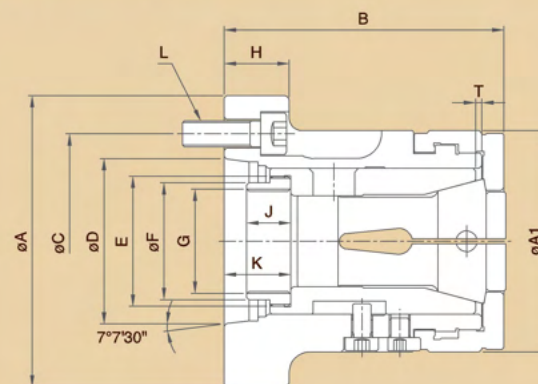
尺寸圖 > Dimensions
