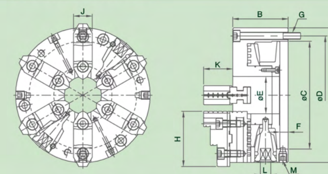
尺寸圖 » Dimensions
