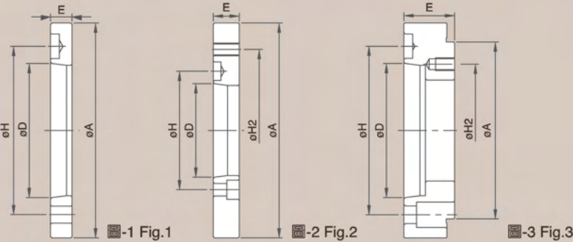
規格表 » Specifications
