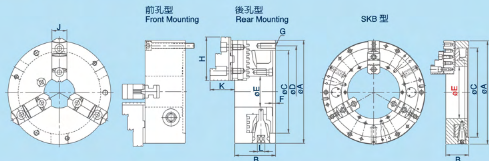
規格表 » Specifications
