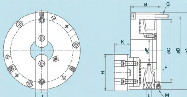
尺寸圖 » Dimensions
