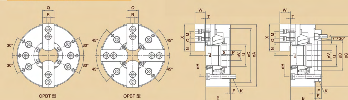
尺寸圖 » Dimensions
