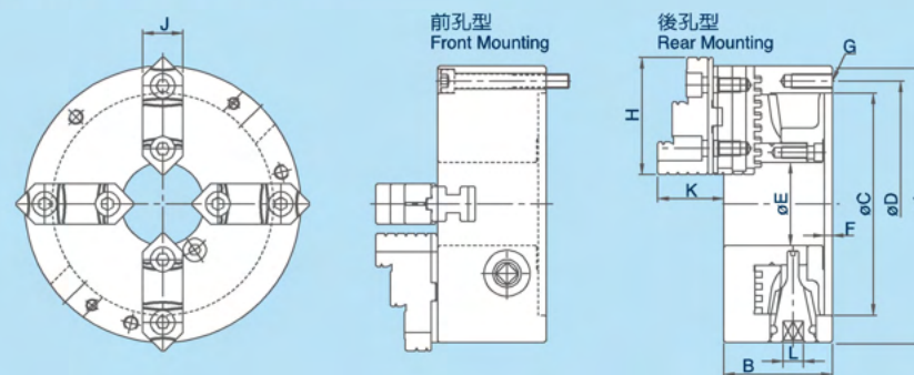
規格表 » Specifications
