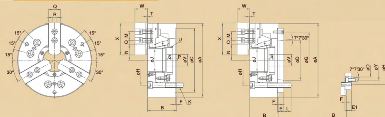
尺寸圖 » Dimensions
