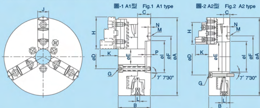
規格表 » Specifications
