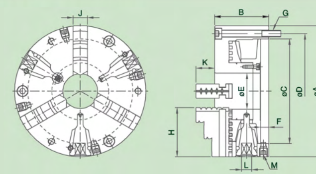
尺寸圖 » Dimensions
