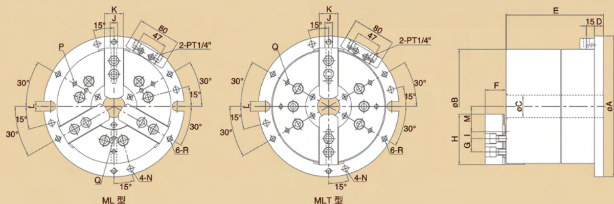
尺寸圖 » Dimensions
