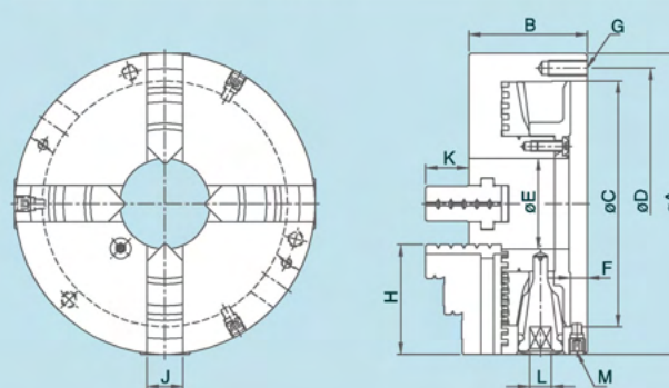
尺寸圖 » Dimensions
