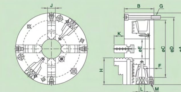
尺寸圖 » Dimensions
