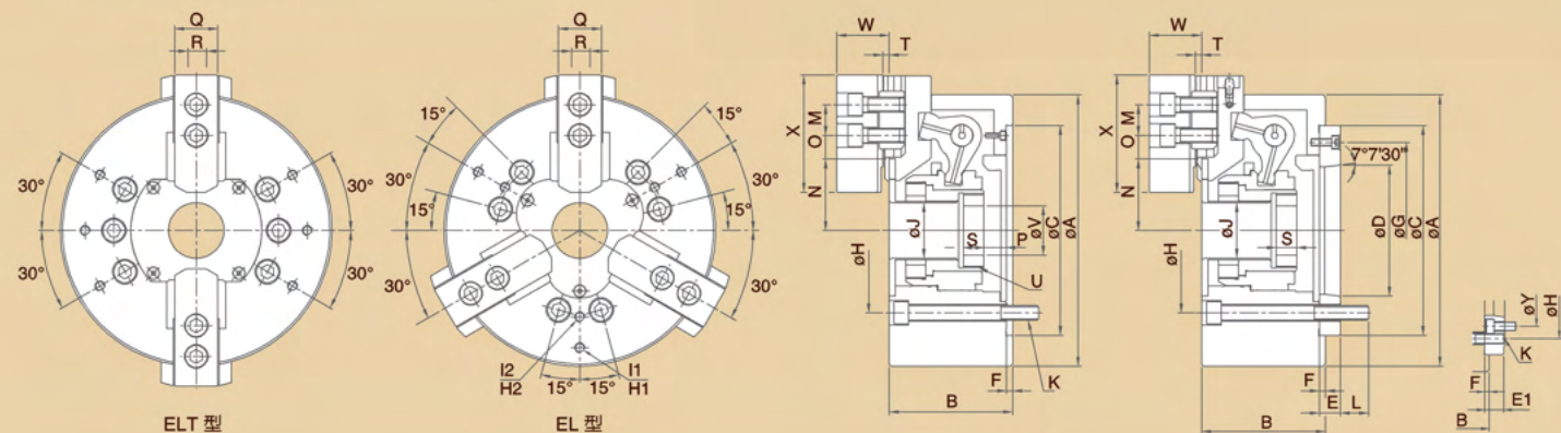
尺寸圖 » Dimensions
