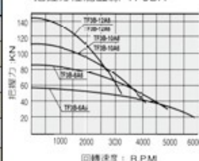
把握力性能曲線 TF3BA
